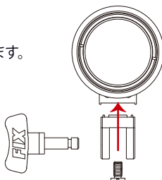
YSベース固定ネジ挿入方向
